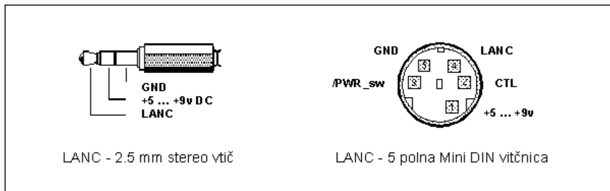
Slika 1 - Razpored priključkov na različnih LANC vtičih
