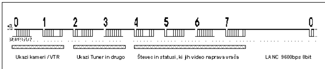
Slika 2 - Blok podatkov, ki se prenaša po LANC protokolu
